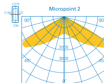
Área aberta (iluminação simétrica)
