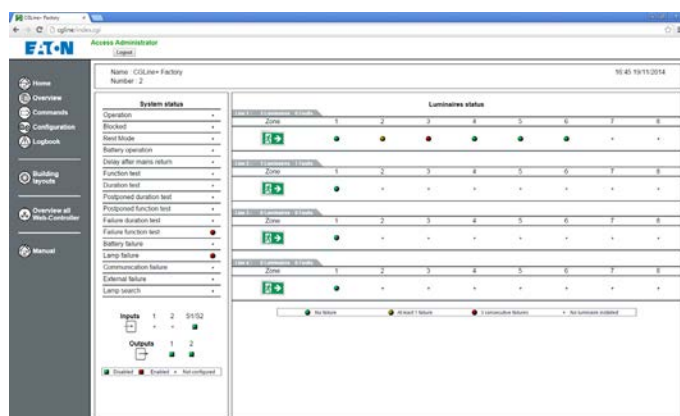
Visualização das zonas na homepage do web server
